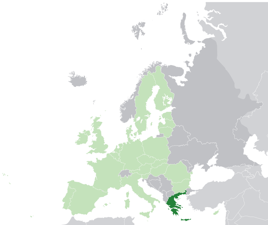
Ilustración 1. Grecia es el país que se muestra en la ilustración en verde oscuro.
